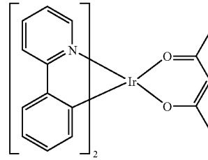
Ir(ppy) 2 (acac)
