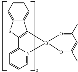
Btp 2 Ir(acac)
