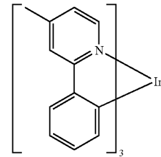
Ir(mppy) 3
