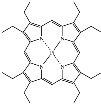
PtOEP
